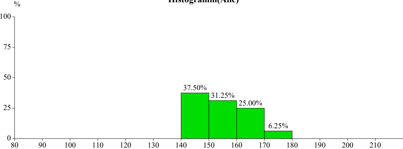
Histogramm(Alle)
